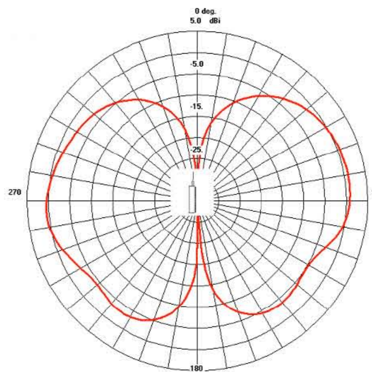
Elevation EXR2400-TNSP
